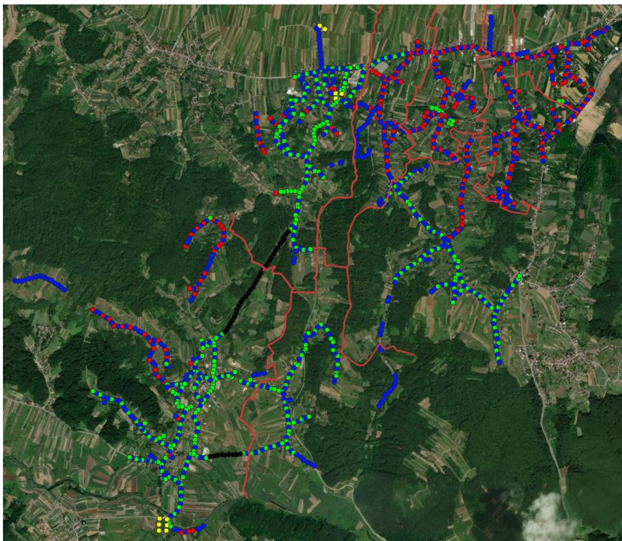
Slika 14. Sustav javne rasvjete na području Općine Sveti Ilija
