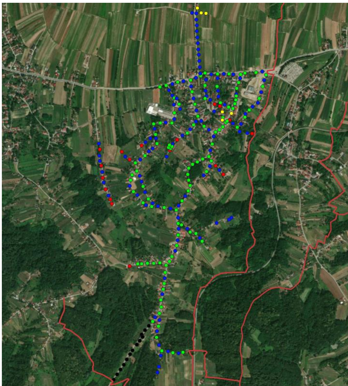
Slika 7. Sustav javne rasvjete na području naselja Sveti Ilija
