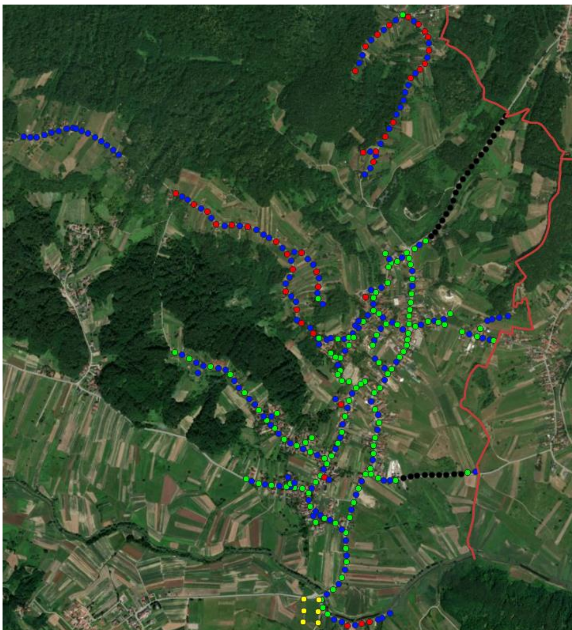
Slika 6. Sustav javne rasvjete na području naselja Beletinec
