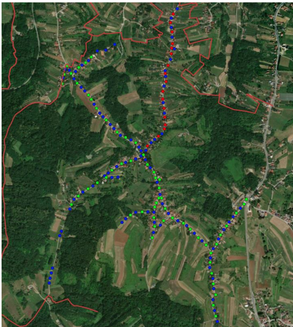
Slika 10. Sustav javne rasvjetе na području naselja Seketin
