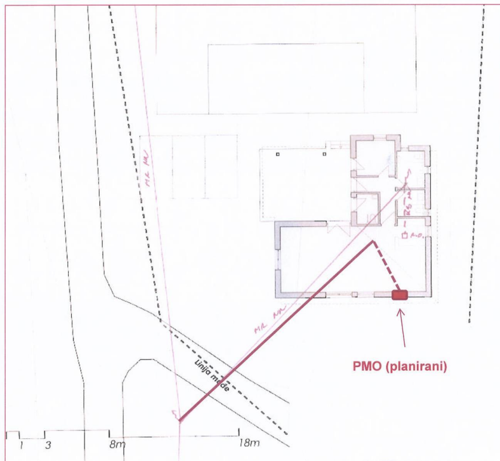
Slika: Prijedlog trase kabelskog voda za priključenje PMO
