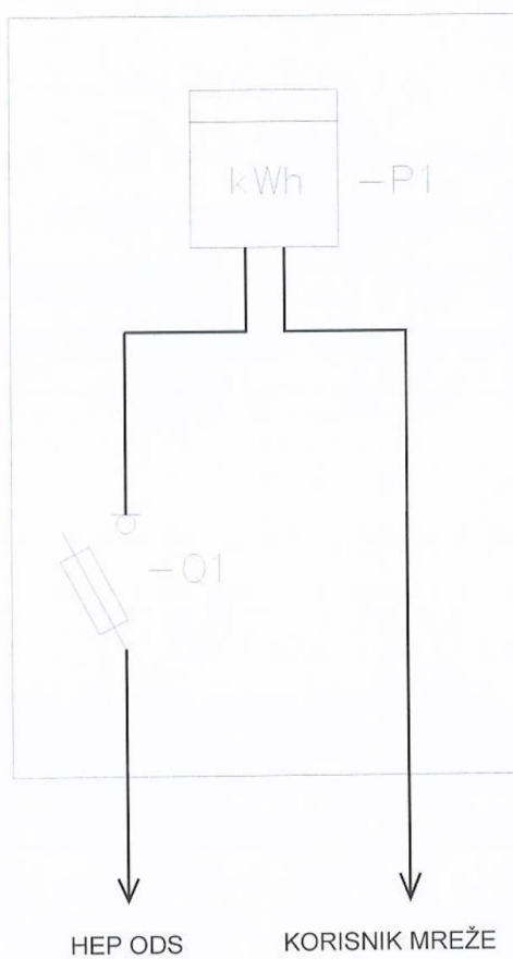
Slika 2. Priključno mjerni ormar (PMO) za 1 OMM - P \leq 50 kW (izravno mjerenje)
